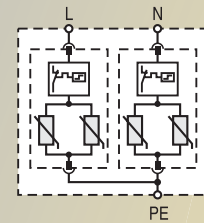
PROTEC B2SR 25/xxx (2+0)
