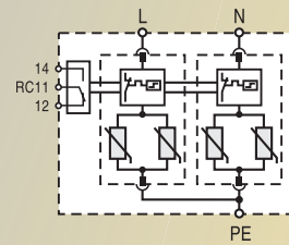
PROTEC B2SR 25/xxx (2+0)
